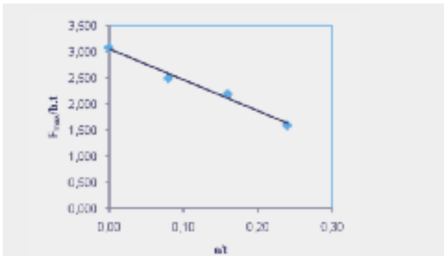
Figuur 3: Draagvermogen in functie van de relatieve excentriciteit van een FOAMGLAS® PERINSUL HL-blok.
