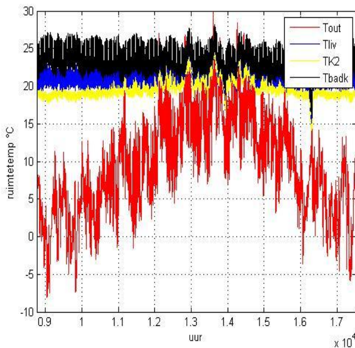
Figuur 51: Ruimtetemperaturen (badk, zwart; living, blauw; slaapkamer, geel) en buitentemp (rood)
