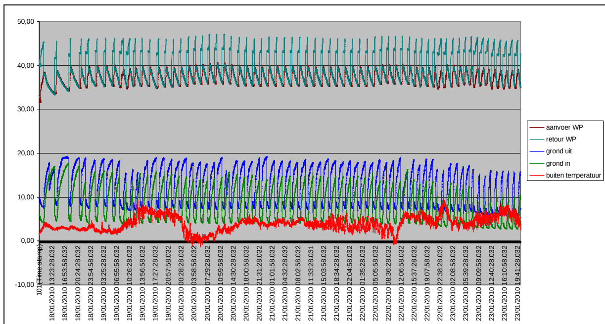
Figuur 24: Aanvoertemperatuur en retour temperatuur ,primair en secundair
